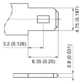
F1 Terminal Unit: mm (inches)
